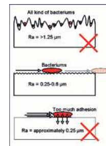
Afbeelding 3 Bij een te glad oppervlak zijn bacteriën moeilijk te verwijderen door onderdruk en adhesie (bron Leser Hamburg).
