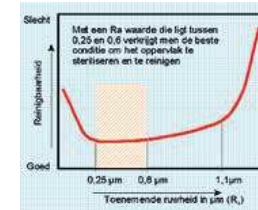
Afbeelding 2 Het reinigen van roestvast staal kan het beste plaatsvinden bij een ruwheid tussen de 0,25 en 0,6 micrometer.
